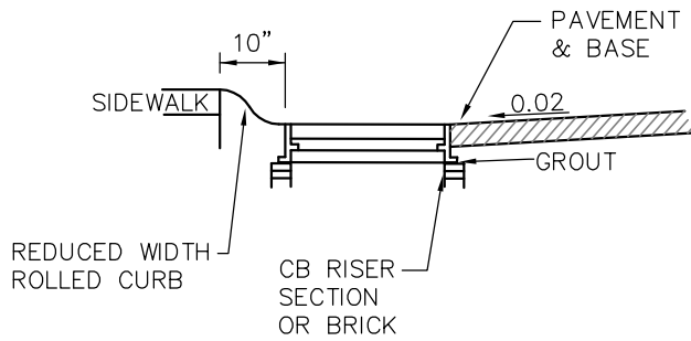
ELEVATION A-A
