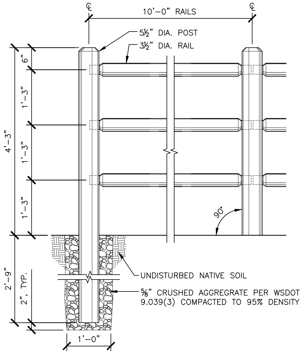
ELEVATION
