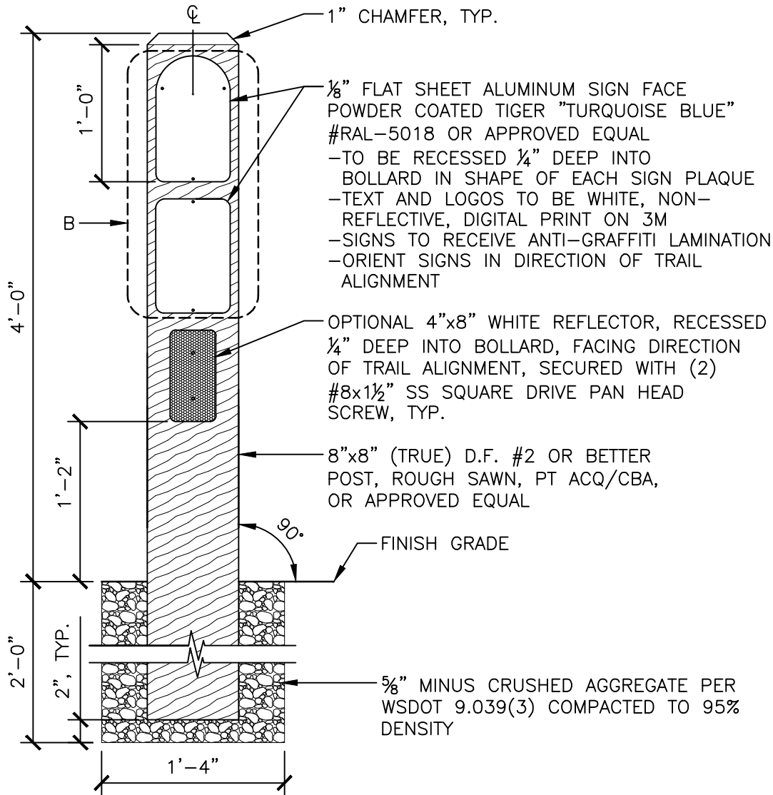
A-BOLLARD DETAIL
